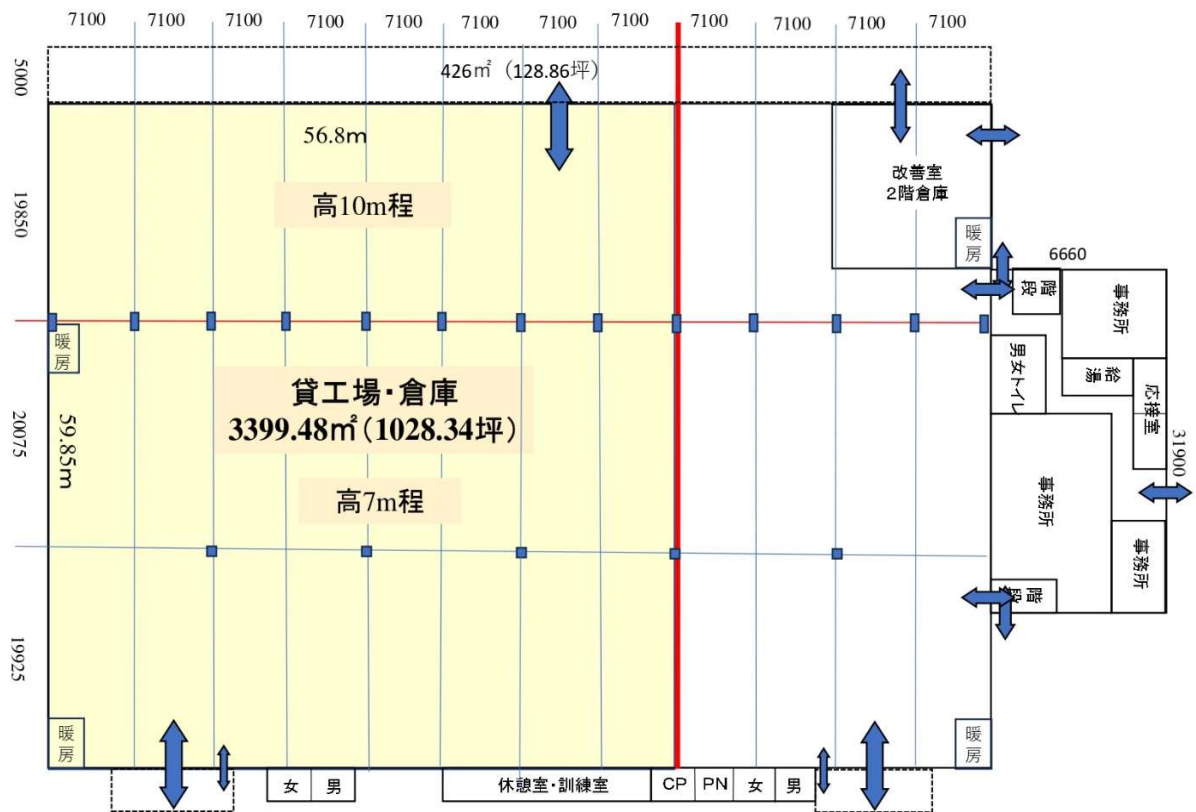
1 階 平面図
